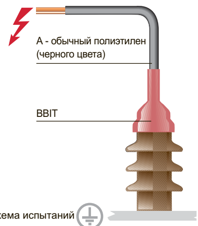
Нетрекинговостойкий материал (трубка черного цвета) разрушается уже после 48 часов испытаний
