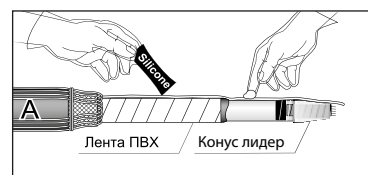
Предварительная парковка стресс-конуса (требуется специальный инструмент)
