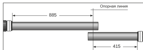
Несимметричная разделка кабеля
