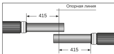
Симметричная разделка кабеля
