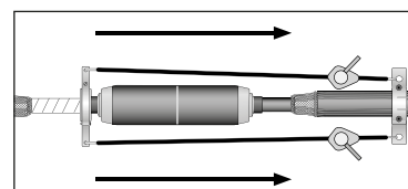
Сборка муфты возможна только с использованием специального инструмента
